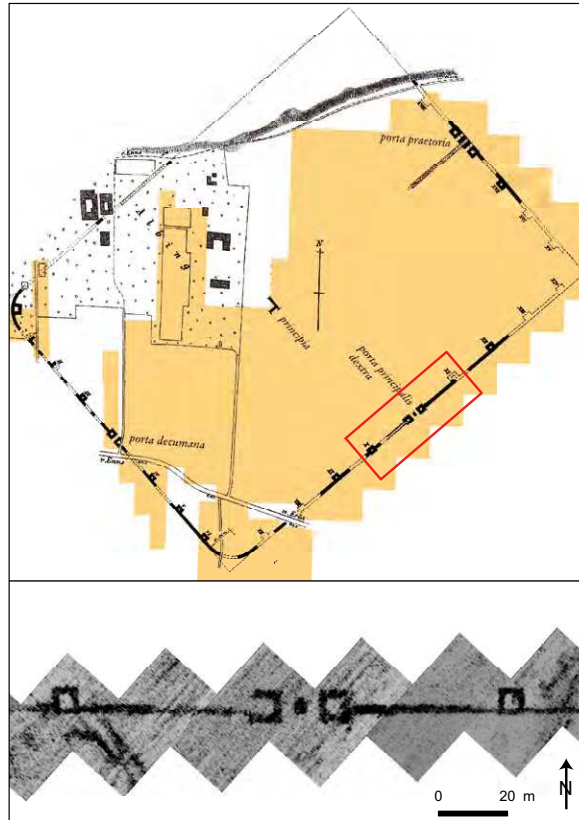
Albing, Messflächen der geophysikalischen Prospektionen im Legionslager. Detail der Messungen an den Fortifikationen des Legionslagers mit Georadar
