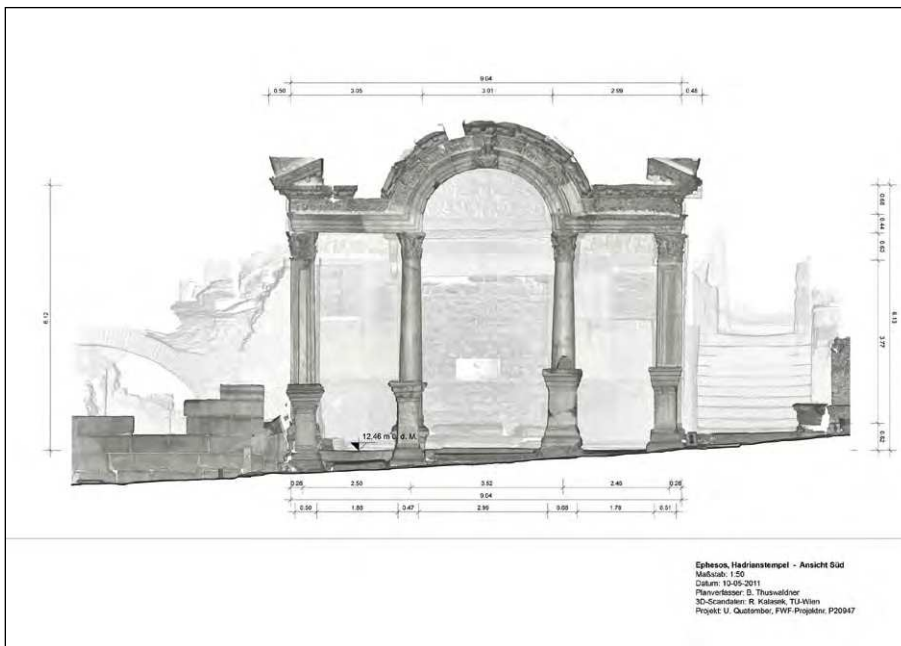
Ephesos, Hadrianstempel. Dokumentation basierend auf den 3-D-Scanning-Daten, Ansicht von Süden (TU Wien, R. Kalasek/B. Thuswaldner)
