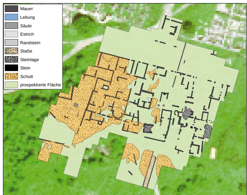
Ephesos, spätantike Wohnbauten in den Verulanushallen. Georadar und interpretiertes Geophysikbild (© ZAMG)
