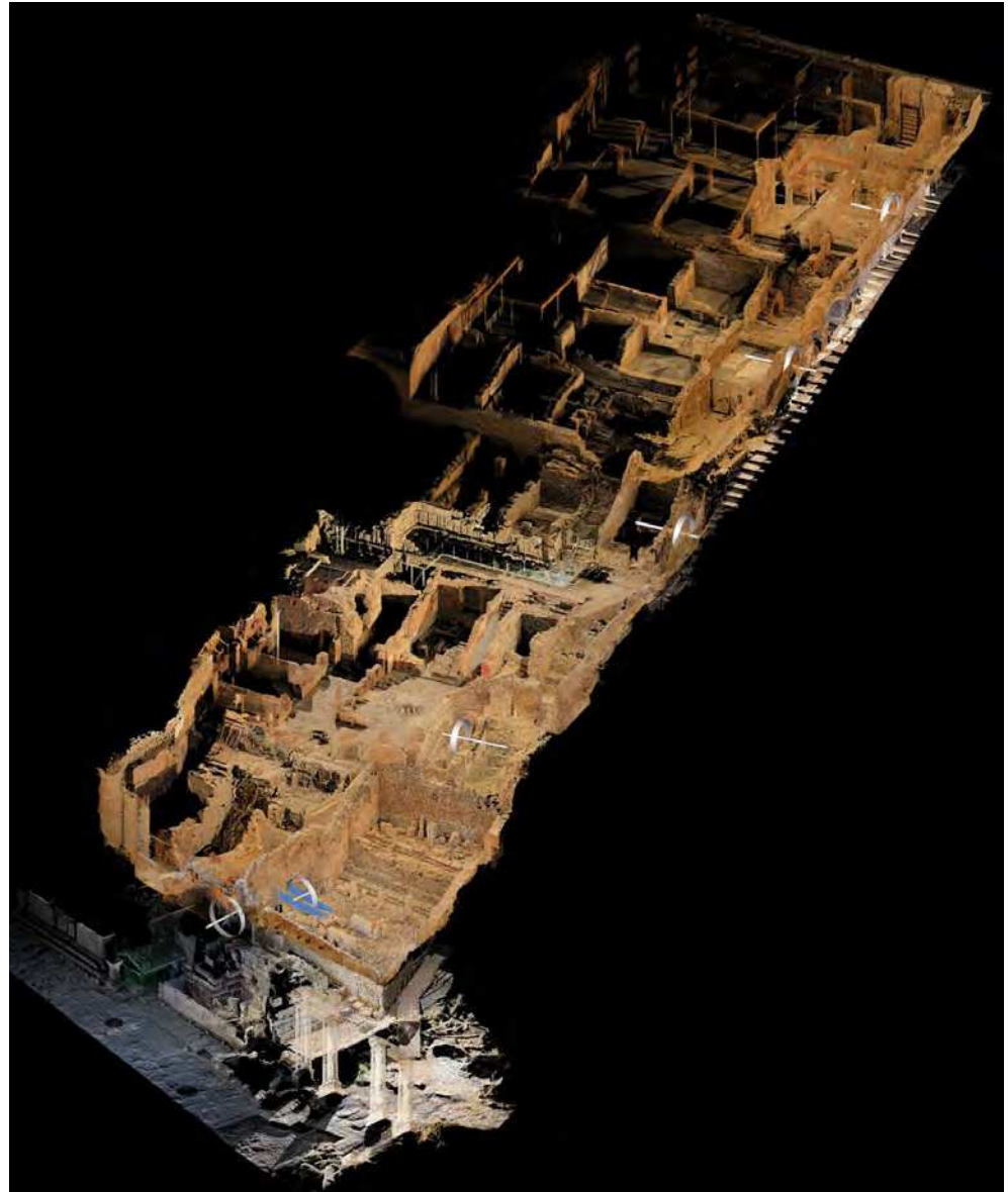
Ephesos, Hanghaus 2. Punktwolke mit Eintragung der Wasserräder (© RGZM Mainz)
