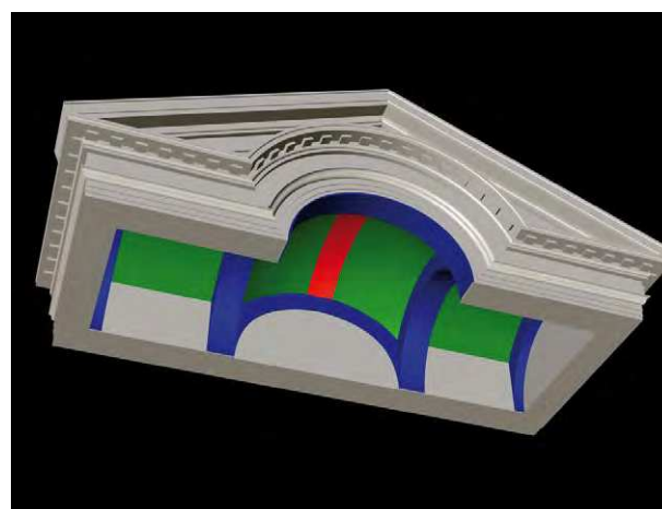
Ephesos, Hadrianstempel. 3-D-Modell der Dachkonstruktion über dem Pronaos (TU Wien, B. Thuswaldner)
