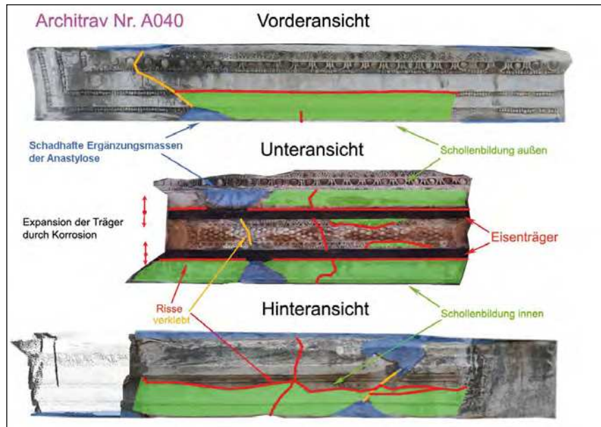
Ephesos, Hadrianstempel. Grafische Darstellung des Schadensbildes von Archi- trav 040A (Foto M. Pliess- nig)
