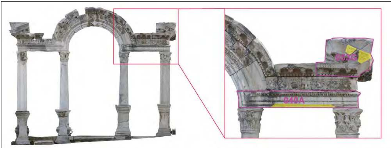
Ephesos, Hadrianstempel. Akut absturzgefährdete Fassadenteile (Architrav 040A, Giebelblock 053G) (Foto M. Pliessnig)
