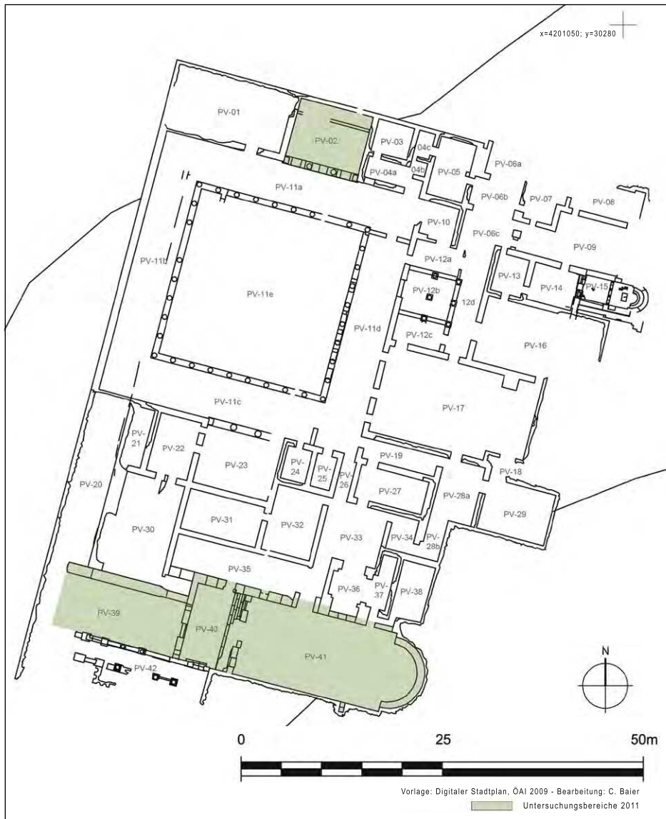
Ephesos, Villenbezirk am Panayırdağ. Generalisierter Grundriss
