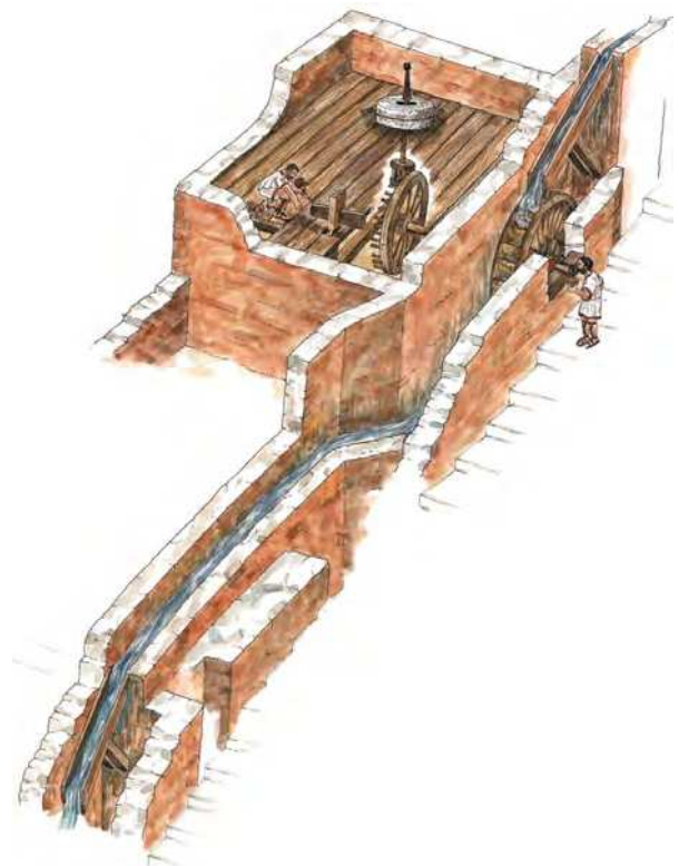
Ephesos, Hanghaus 2, byzantinische Werkstätten. Rekonstruktion einer byzantinischen Mühle (© RGZM Mainz)
