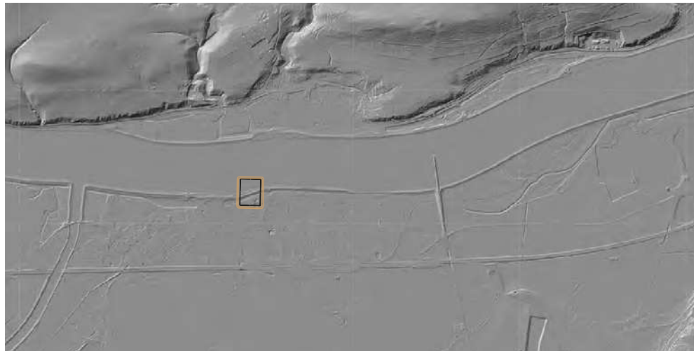
Arelape-Pöchlarn, digitales Höhenmodell der Umgebung des Auxiliarkastells. M 1 : 4.000 (Kartengrundlage © GEOinfo Niederösterreich, Karte S. Schmid)
