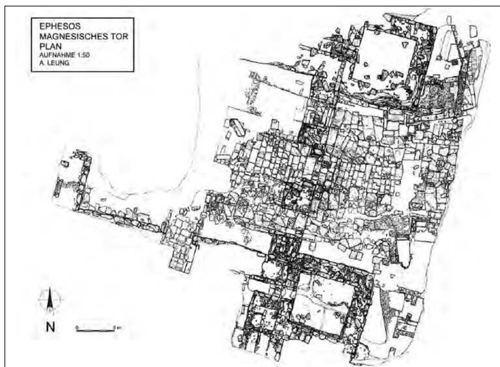
Ephesos, Magnesisches Tor. Steingerechter Grundrissplan (A. Leung)
