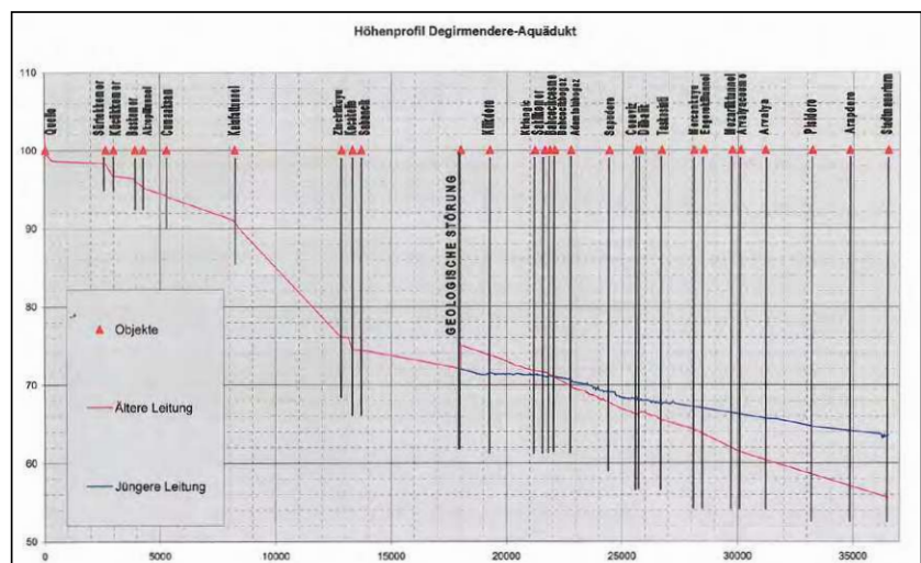
Ephesos, Değirmendere-Aquädukt. Höhenprofil des Aquädukts mit Doppelleitung (Grafik C. Kurtze/E. Unger)
