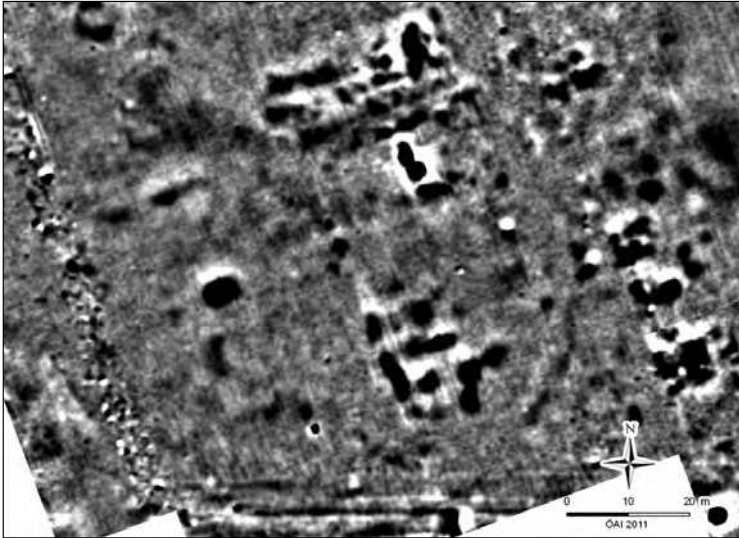
Aquileia, geophysikalische Messungen mit Magnetik im Bereich der Porta triumphalis im halbrunden Südausschluss des Circus (Ausschnitt)
