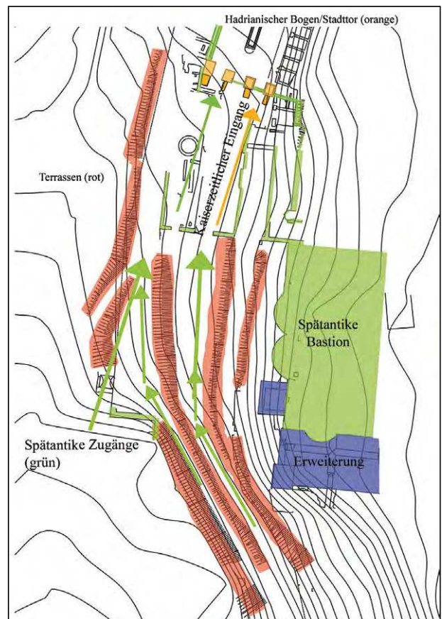
Antiochia in Pisidien, südwestliche Befestigungswerke mit Stadttor, Bastion und Terrassen
