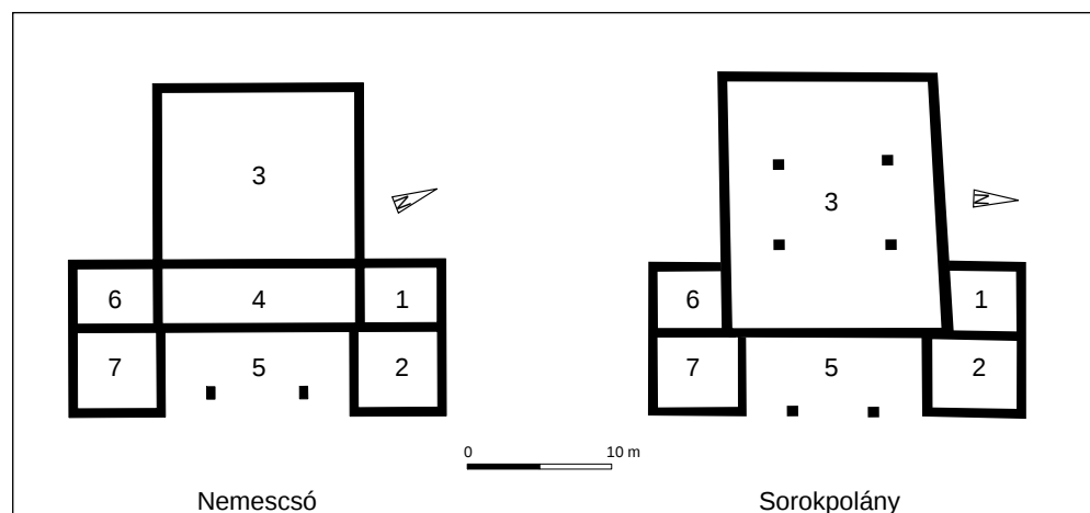
Die Grundrisse der Straßenstationen von Nemescsó und Sorokpolány
