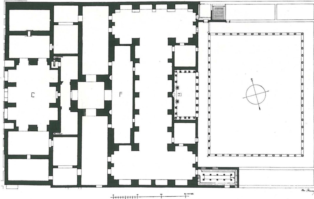
12: Stadiathermen; vorläufige Grundrißskizze.
